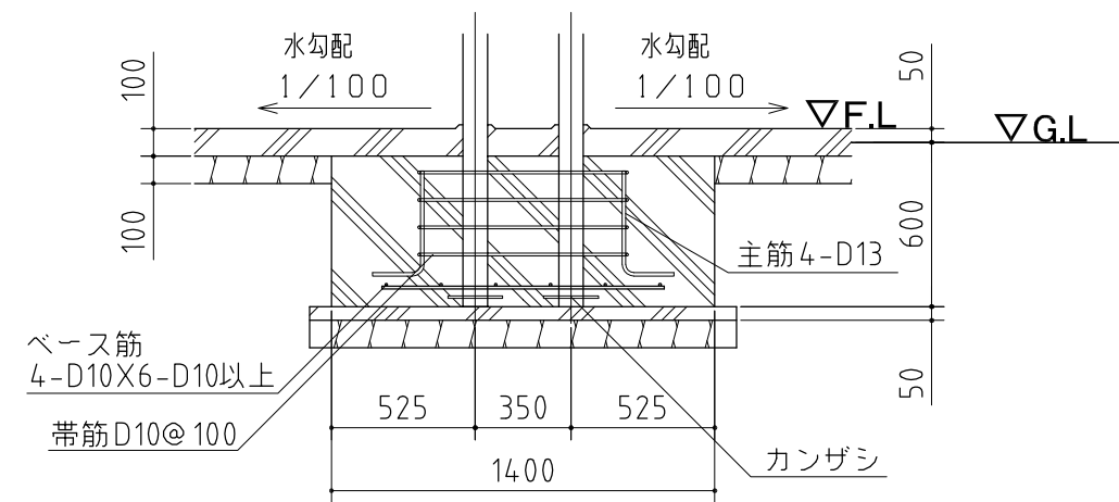
A-A' 断面
